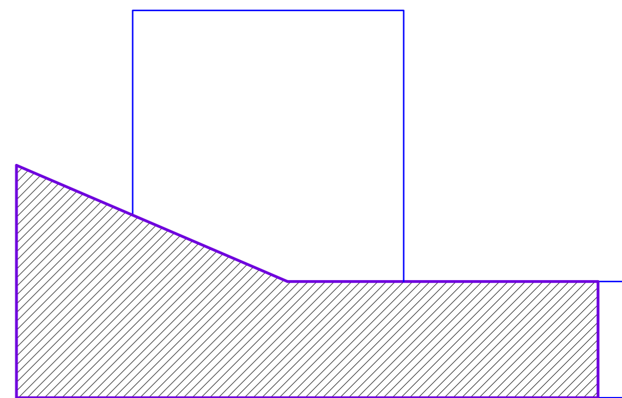
COUPE B-B'
